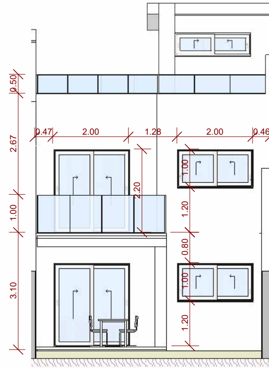
8 2 Alzado Norte 08 1 : 100
