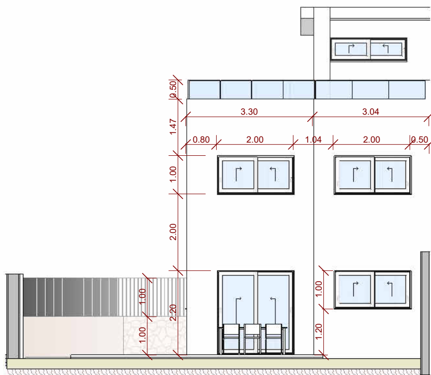
8 1 Alzado Norte 09 1 : 100
