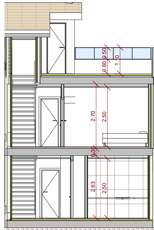
ST Sección Transversal 08 1 : 100
