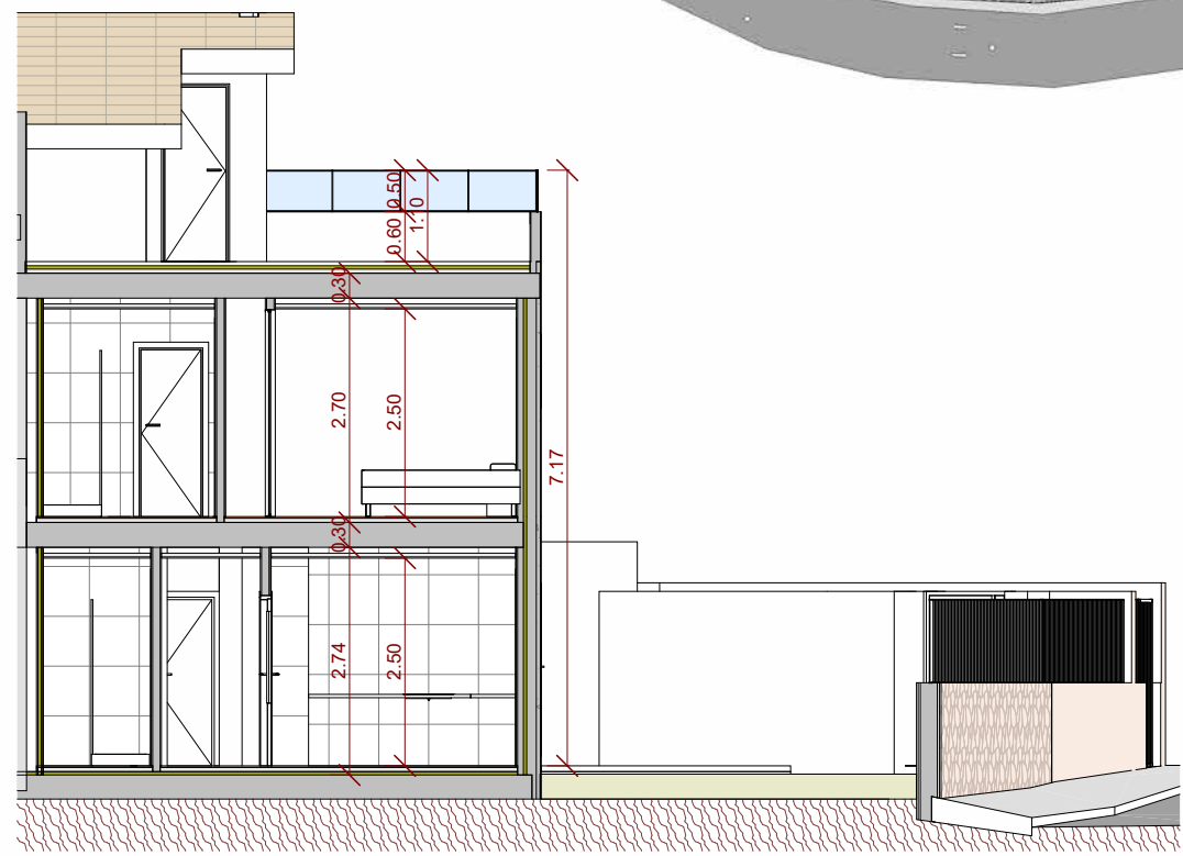
ST Sección Transversal 09 1 : 100
