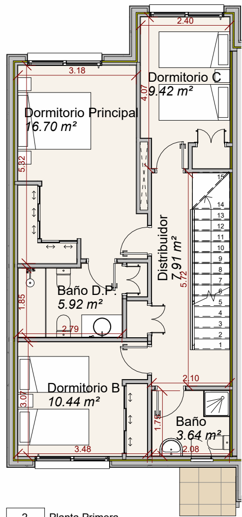
2 Planta Primera 07 1 : 100
