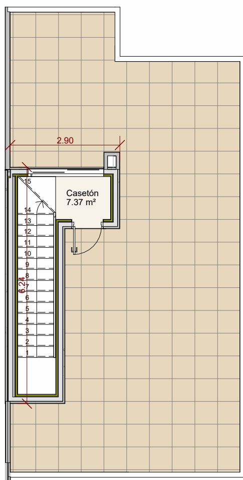
3 Planta Cubierta 09 1 : 100
