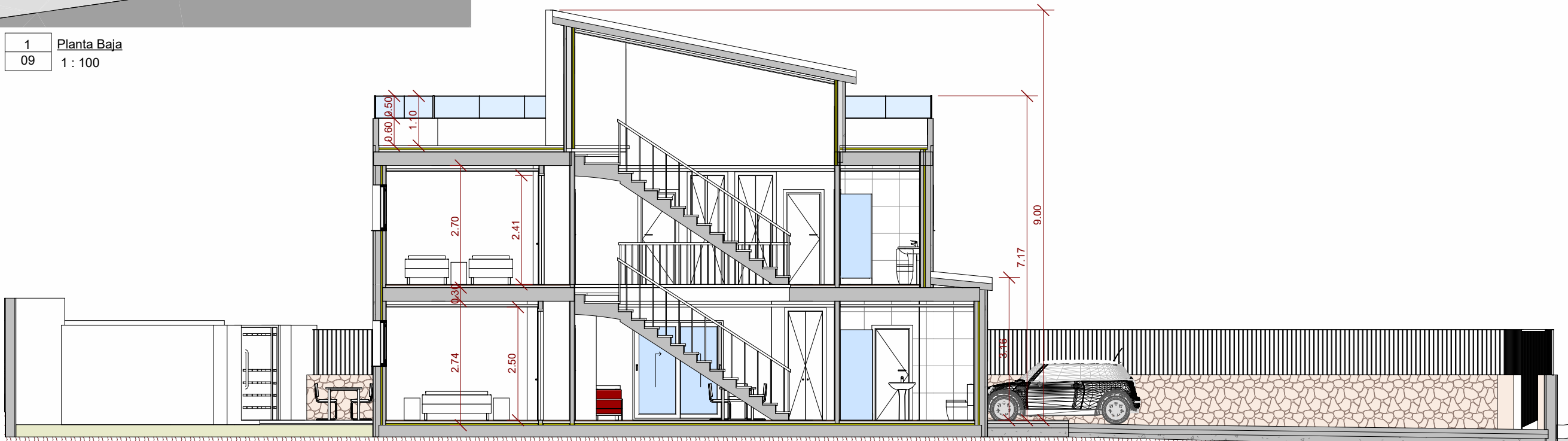
SL Sección Longitudinal 09 1 : 100
