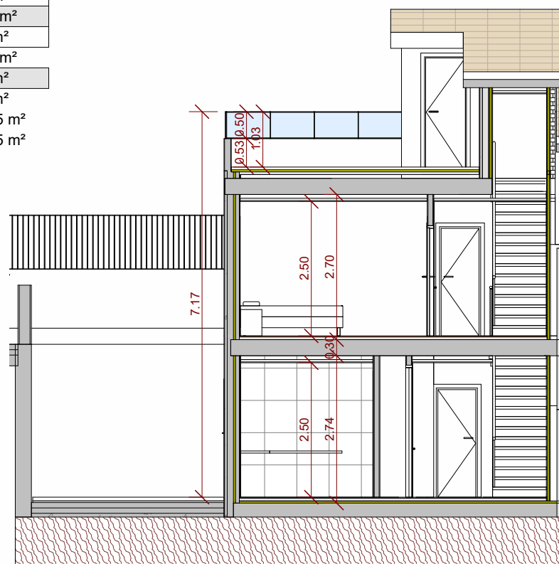
ST Sección Transversal 07 1 : 100
