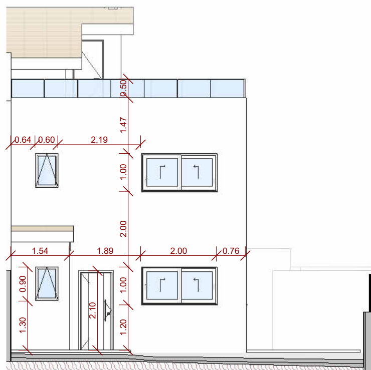
9 1 Alzado Sur 09 1 : 100
