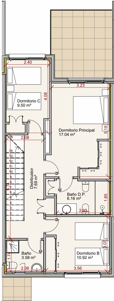
2 Planta Primera 08 1 : 100
