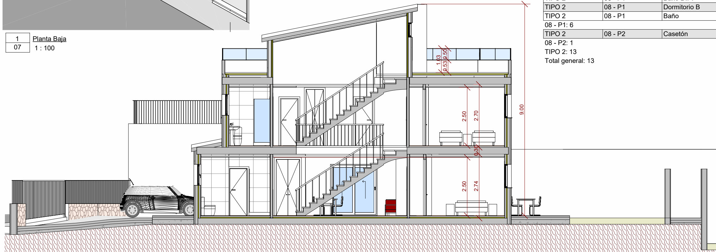
SL Sección Longitudinal 07 1 : 100
