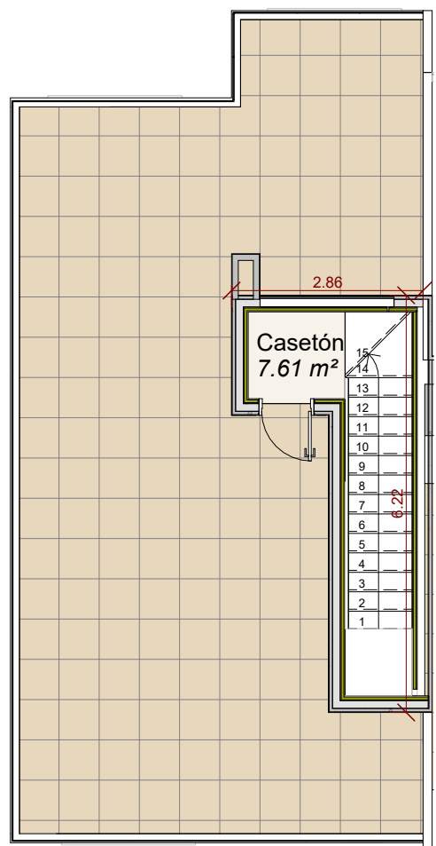
3 Planta Cubierta 07 1 : 100
