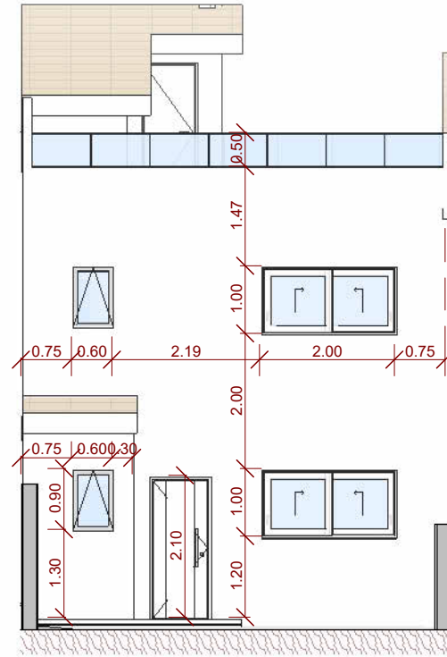
9 2 Alzado Sur 08 1 : 100
