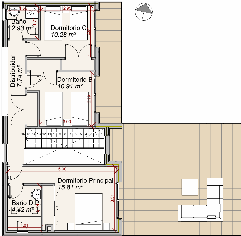
2 06 Planta Primera 1 : 100
