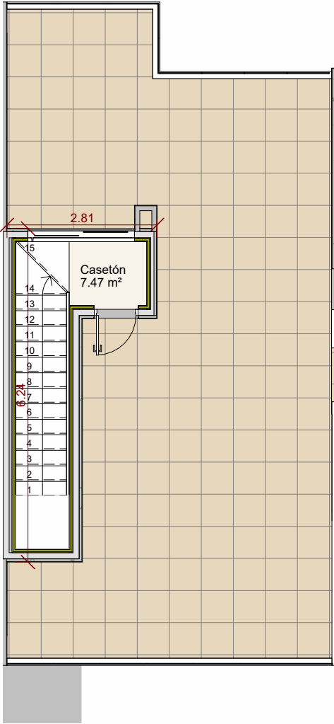
3 Planta Cubierta 08 1 : 100
