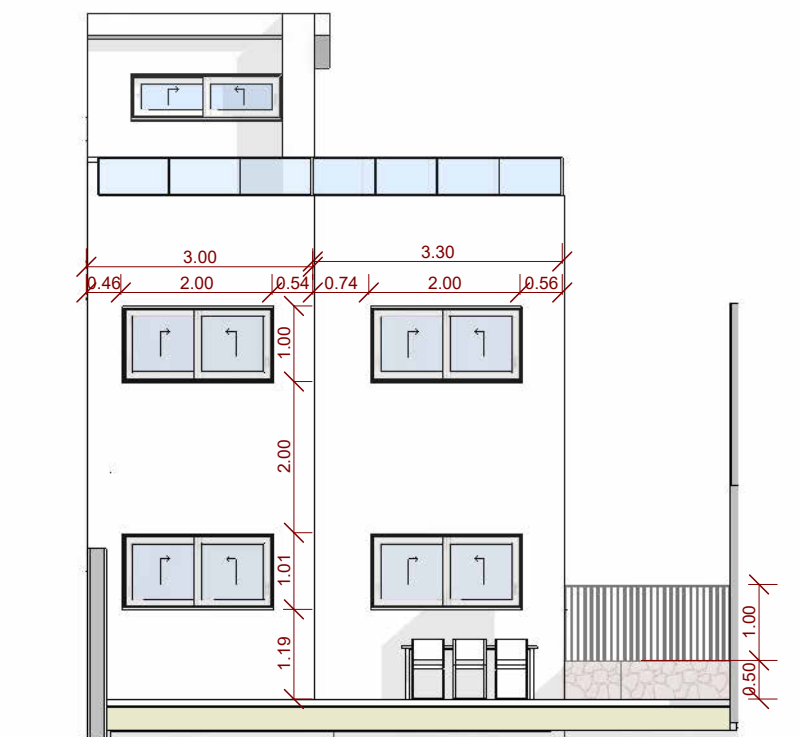
8 Alzado Norte 07 1 : 100
