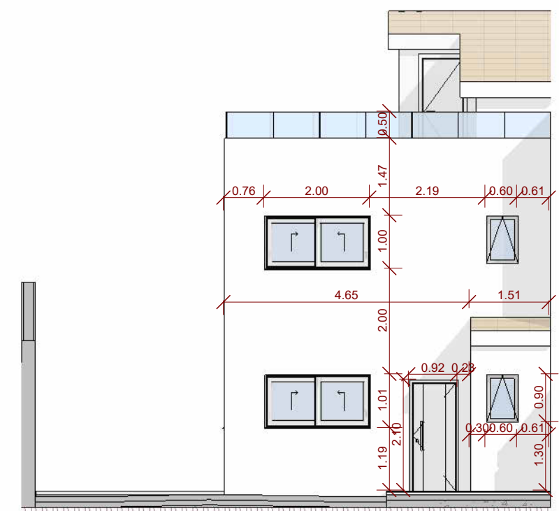
9 Alzado Sur 07 1 : 100
