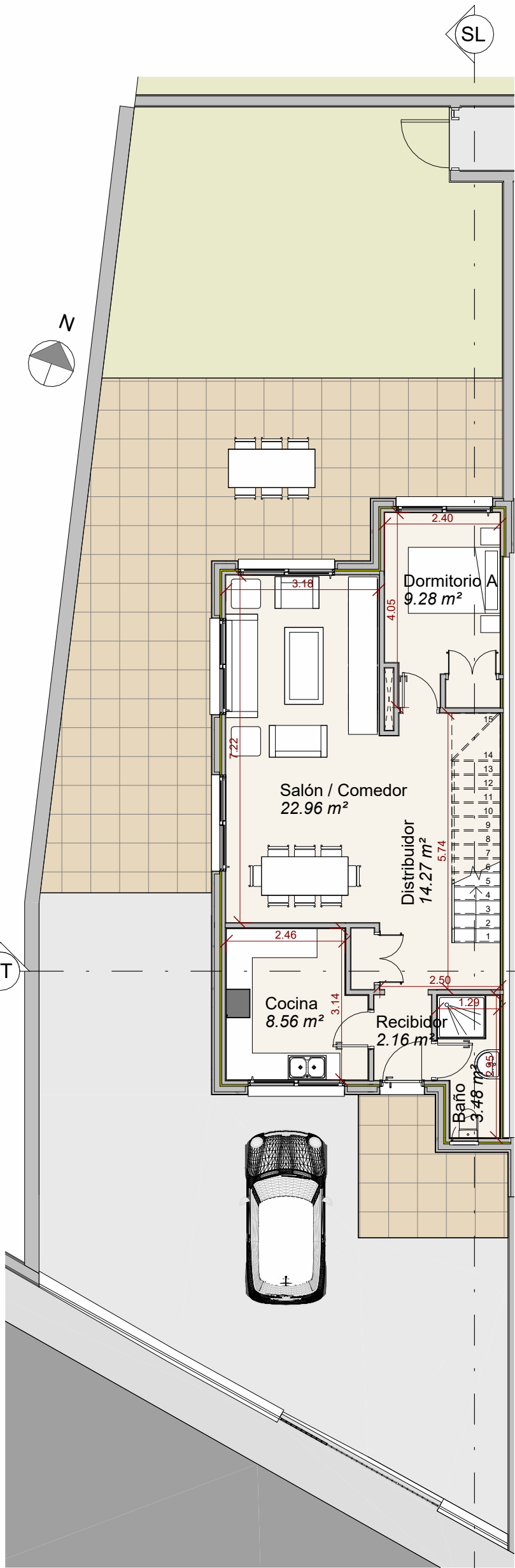
1 Planta Baja 07 1 : 100
